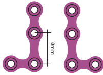
2.0mm L-Plate, Type-III, 90°
