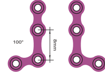
2.0mm L-Plate, 100°
