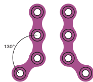
2.0mm L-Plate, 130°
